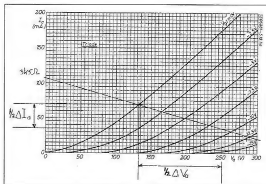
fig.25 Optimale belasting pseudo-triode.
